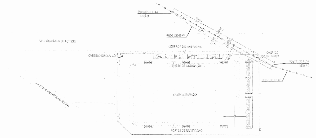
Planta Baixa de Situação do Centro Esportivo
