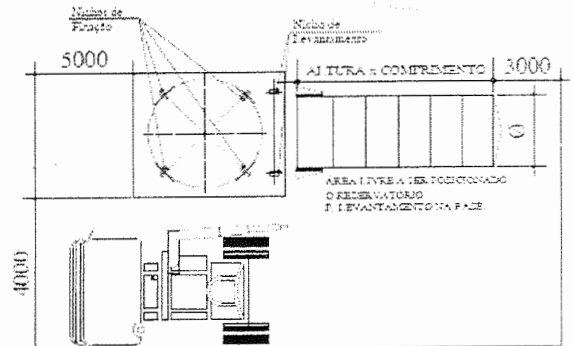
VISTA SUPERIOR IÇAMENTO DO RESERVATÓRIO
