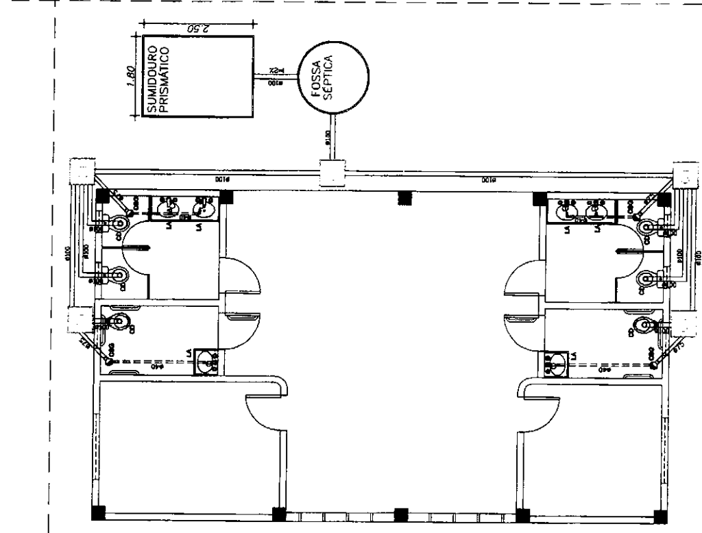
01 PLANTA BAIXA - SANITÁRIA ESCALA: 1/75
