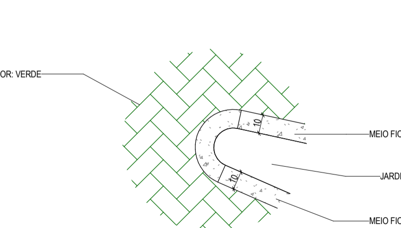
6 DETALHE 04 - SETOR B ESCALA 1:20
