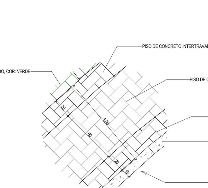
3 DETALHE 03 - SETOR B ESCALA 1:20
