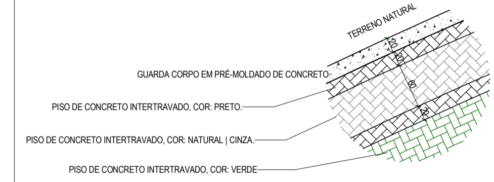
4 DETALHE 02 - SETOR C 1 : 50
