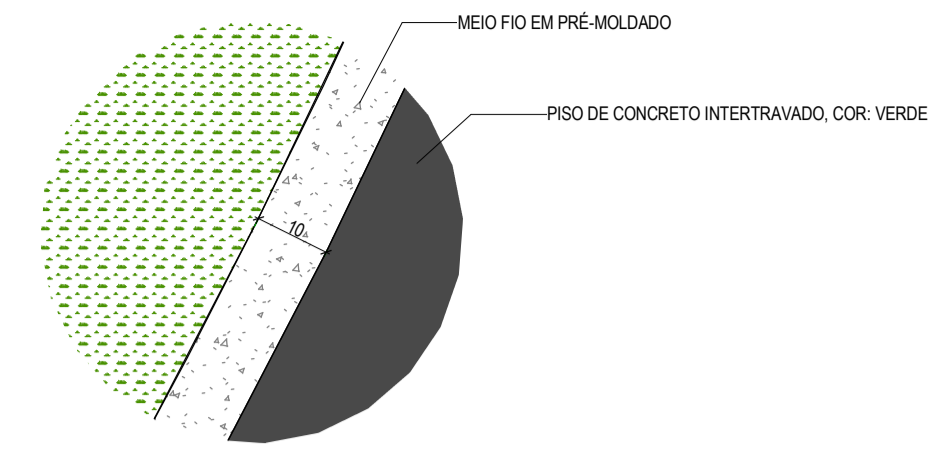
3 DETALHE 03 - SETOR C 1 : 10
