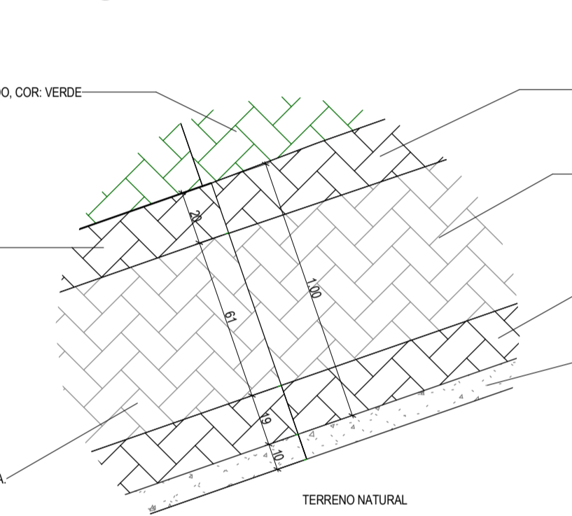
5 DETALHE 01 - SETOR B ESCALA 1:10
