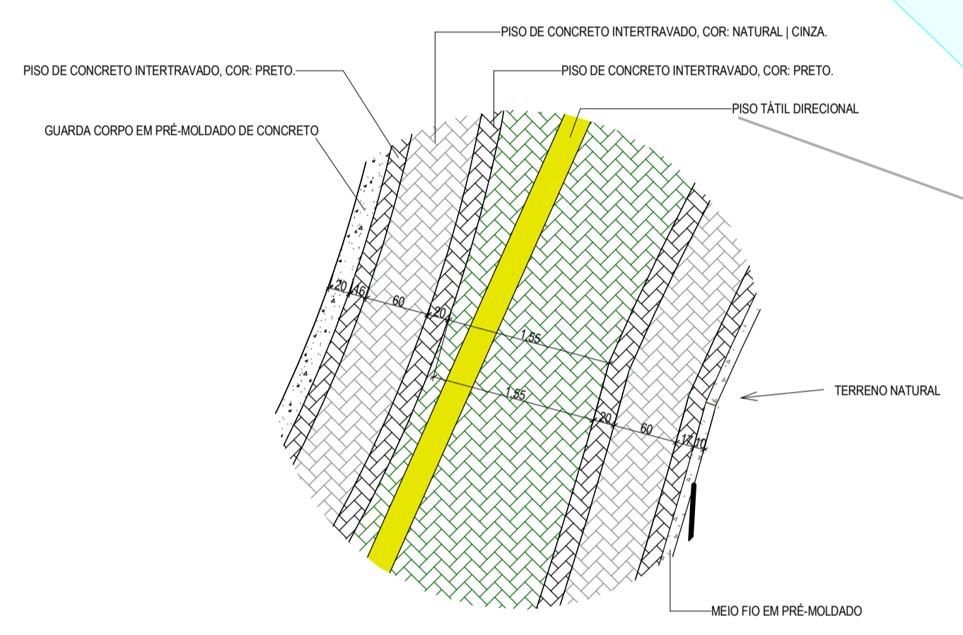
5 DETALHE 01 - SETOR C 1 : 50
