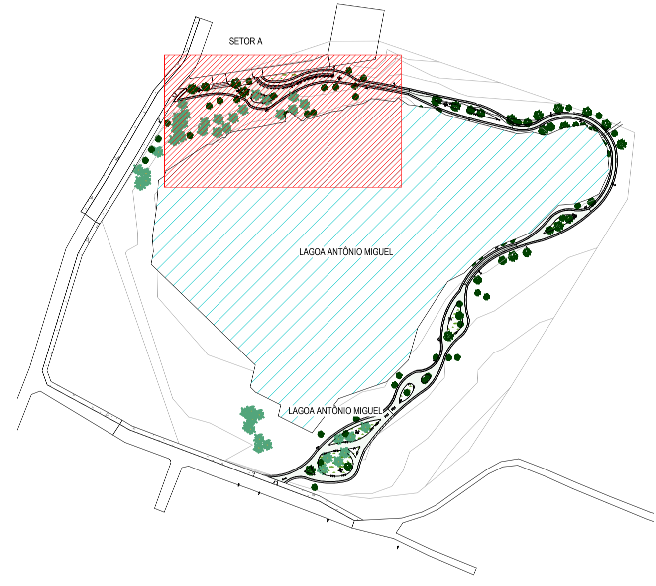
2 PLANTA CHAVE DE PAISAGISMO - SETOR A ESCALA 1:2000
