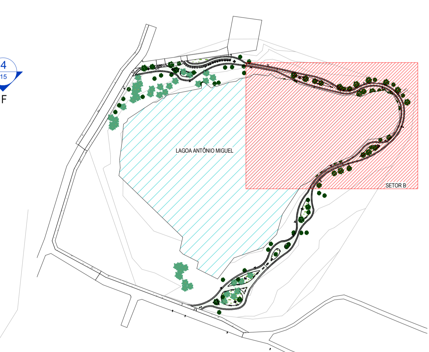
2 PLANTA AP CHAVE SETOR B ESCALA 1:2000
