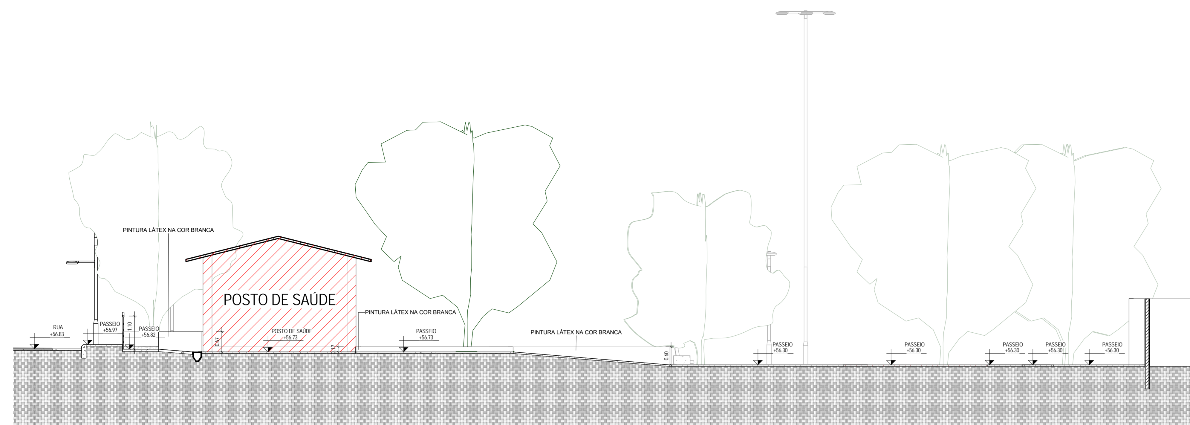
1 CORTE A-A 1:75
