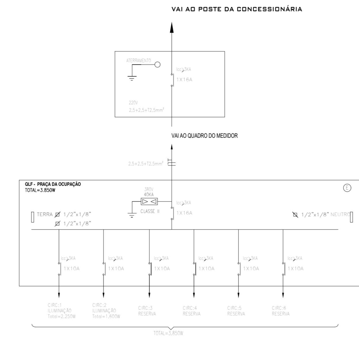
4 DIAGRAMA UNIFILAR - QLF 1:100
