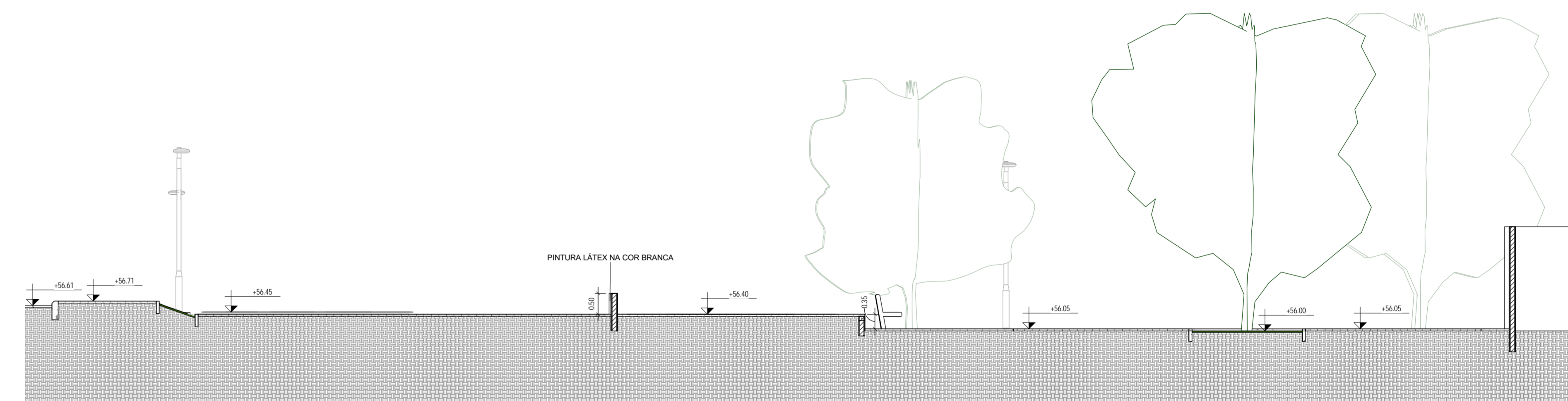
4 CORTE D-D 1:75
