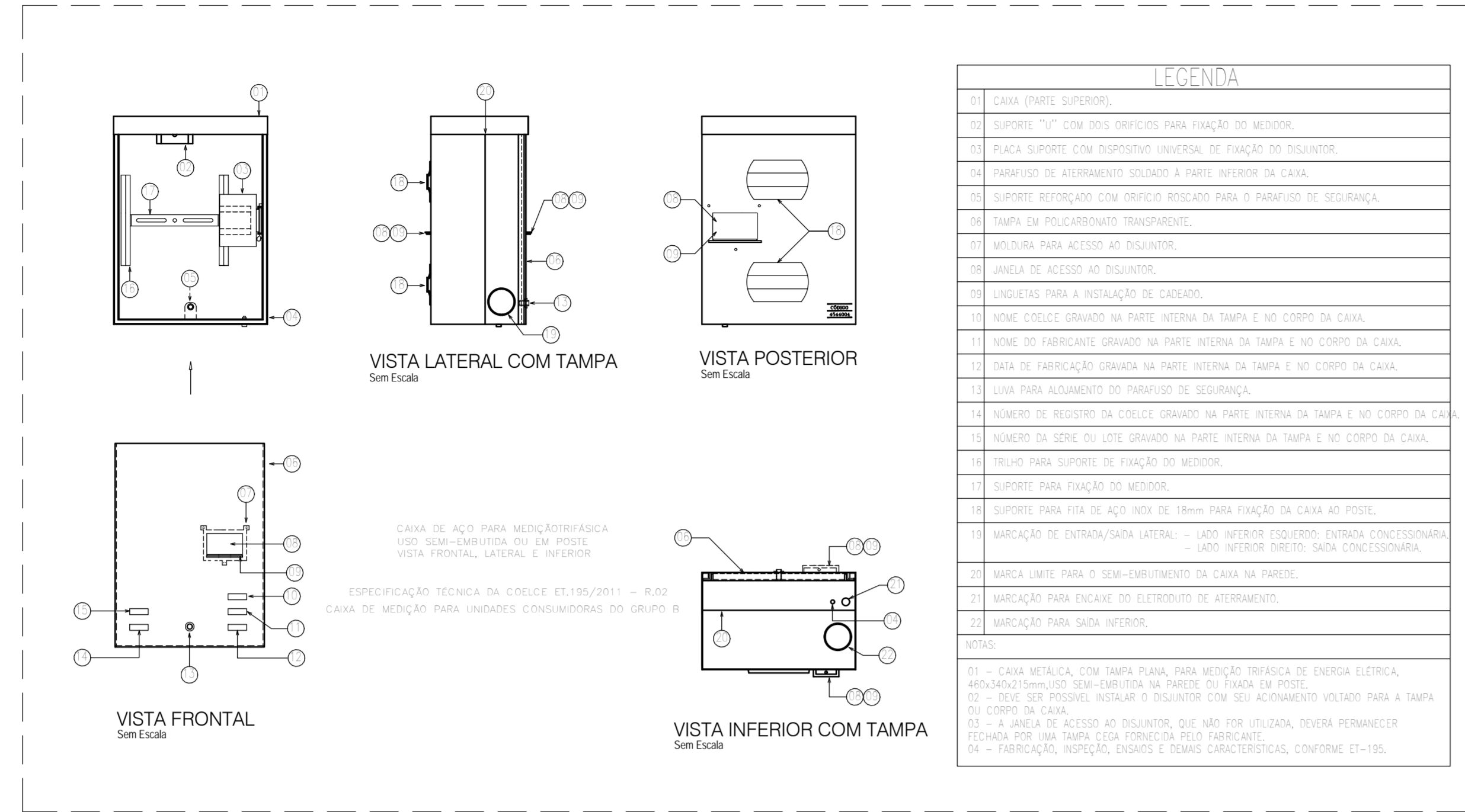
1 Detalhe Caixa de Medição 1:10
