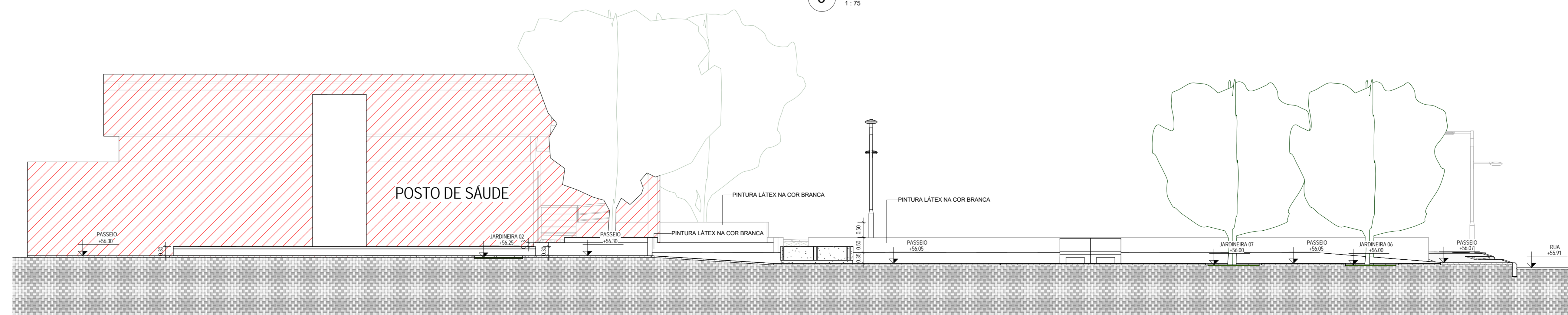
4 CORTE I-I 1:75
