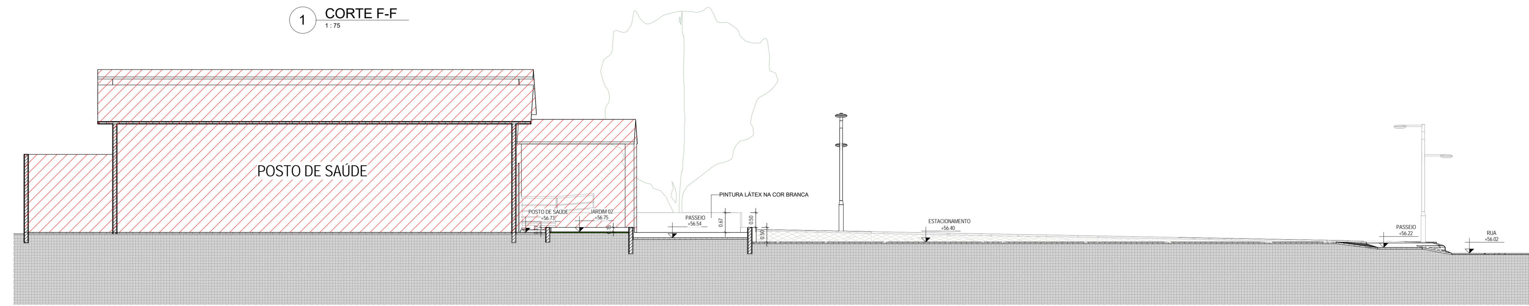
2 CORTE G-G 1:75
