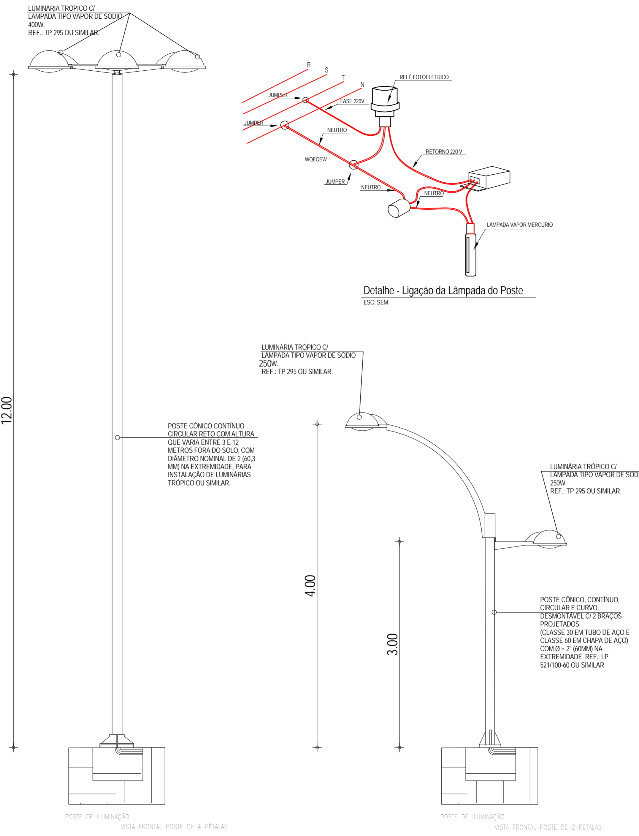
2 Detalhe Poste de Urbanização 1:30
