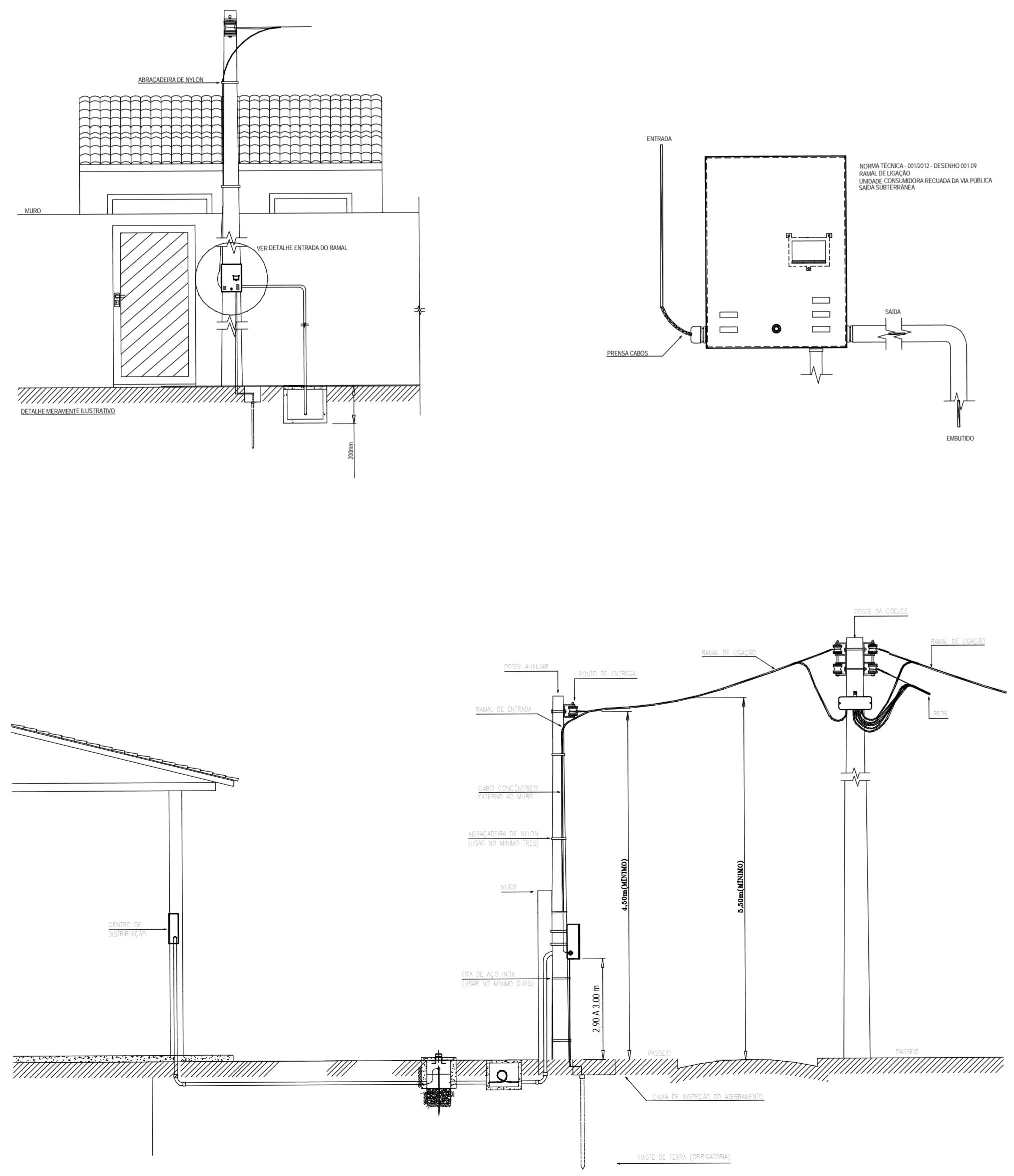
5 DETALHES ELÉTRICOS 1:75
