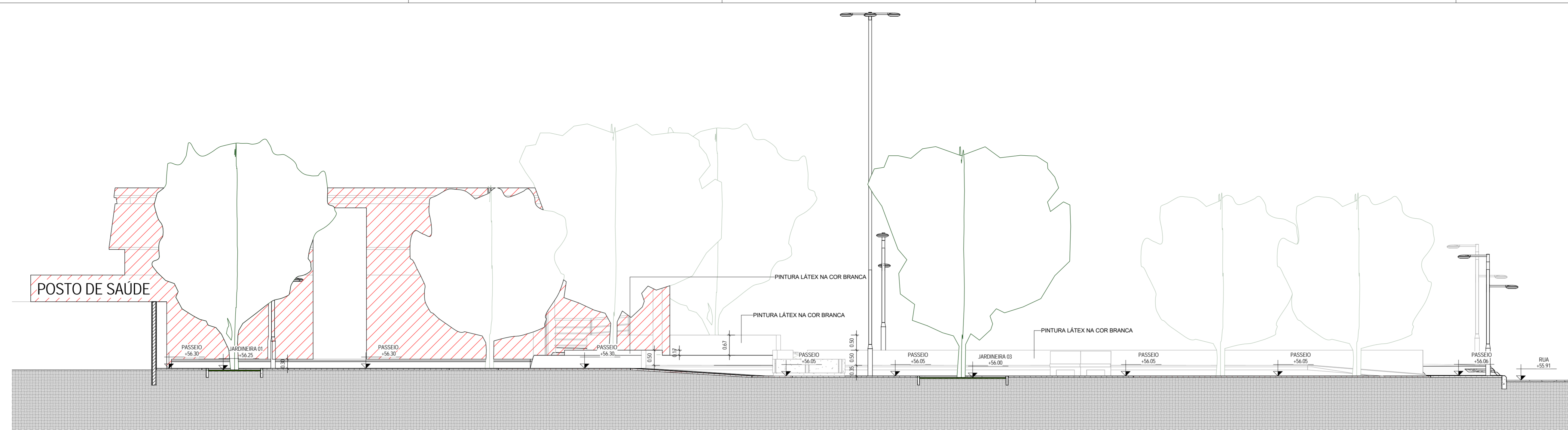
1 CORTE J-J 1:75
