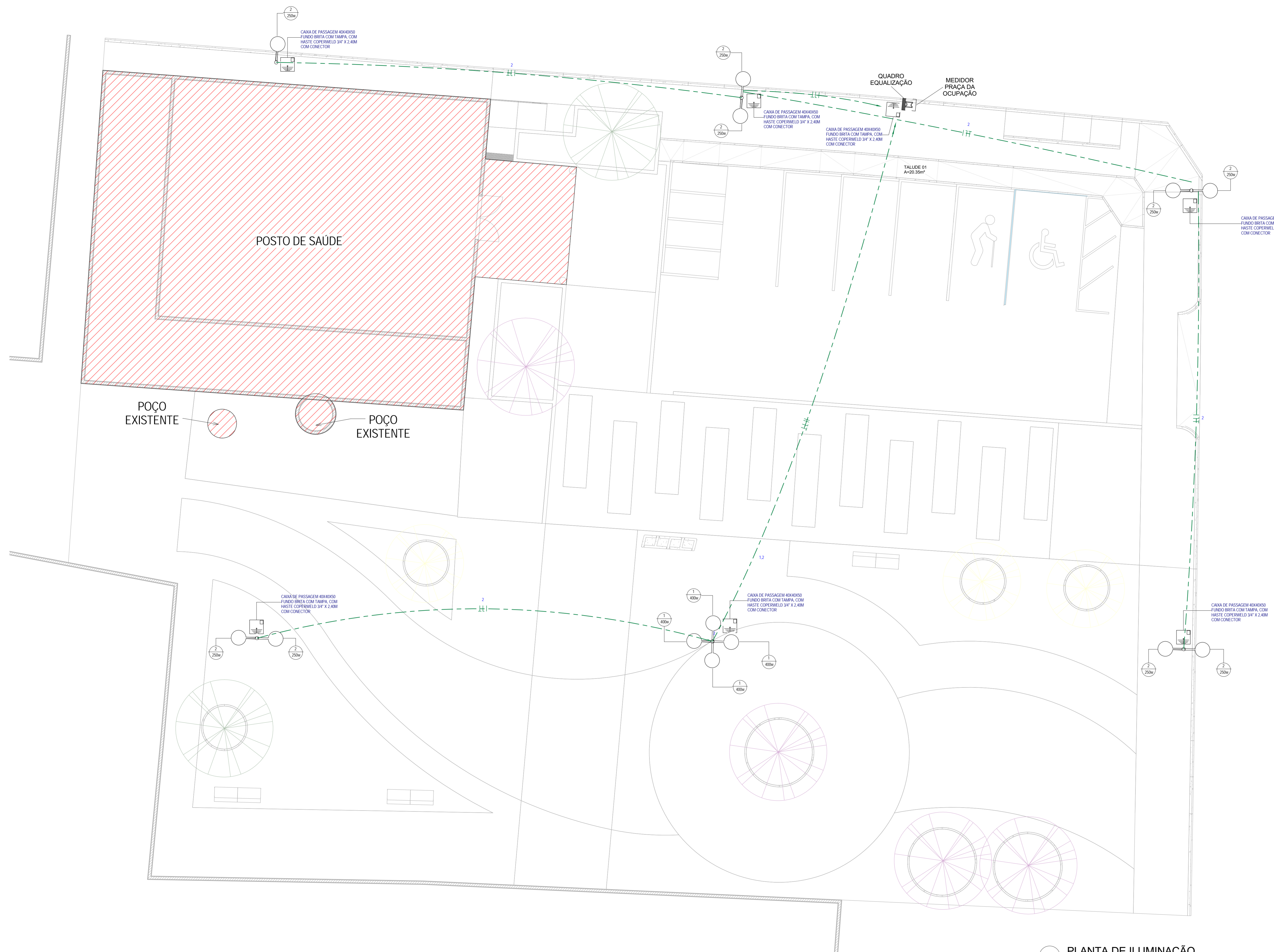
1 PLANTA DE ILUMINAÇÃO 1:75
