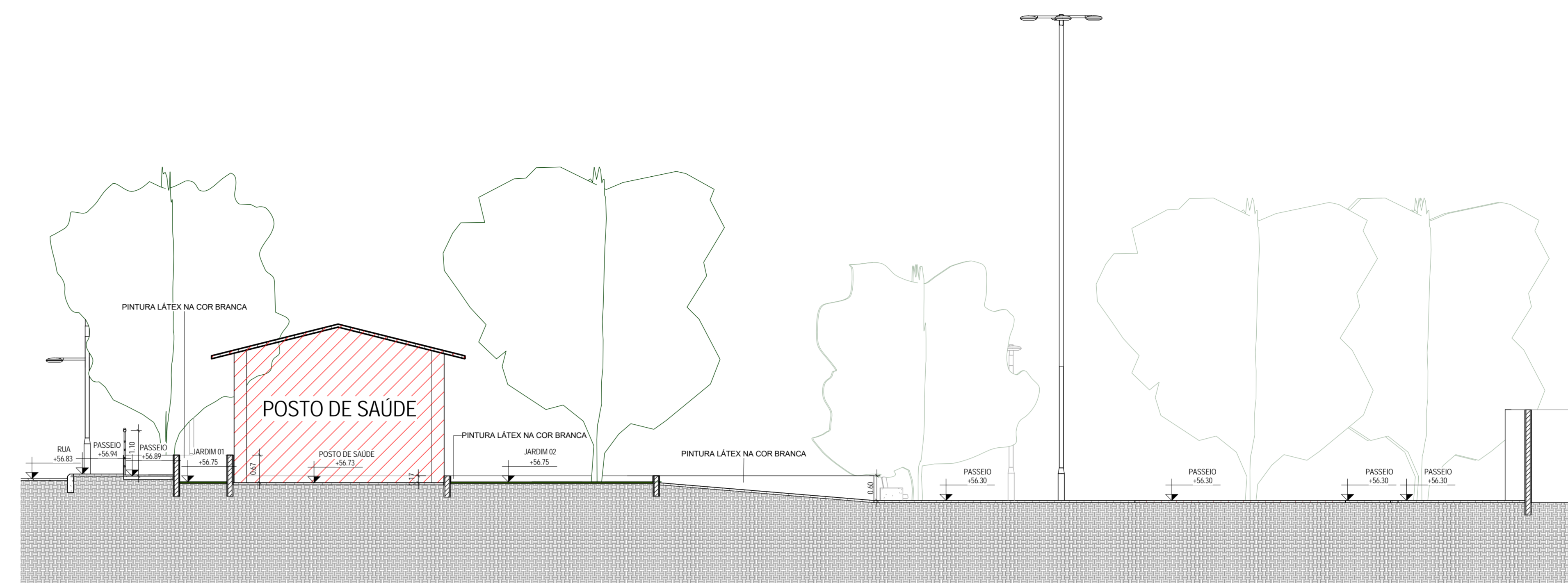
2 CORTE B-B 1:75
