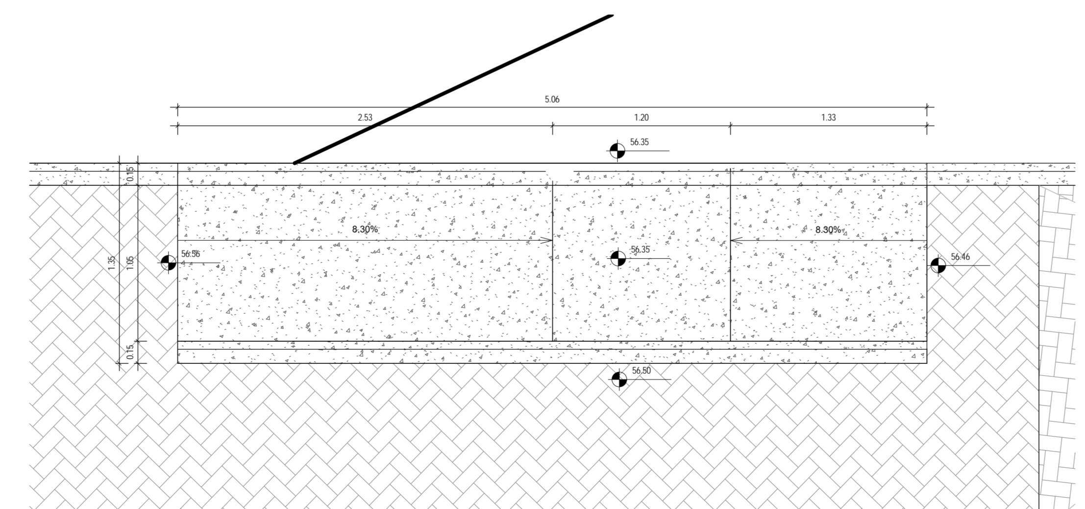
3 DETALHE DA RAMPA 1:25
