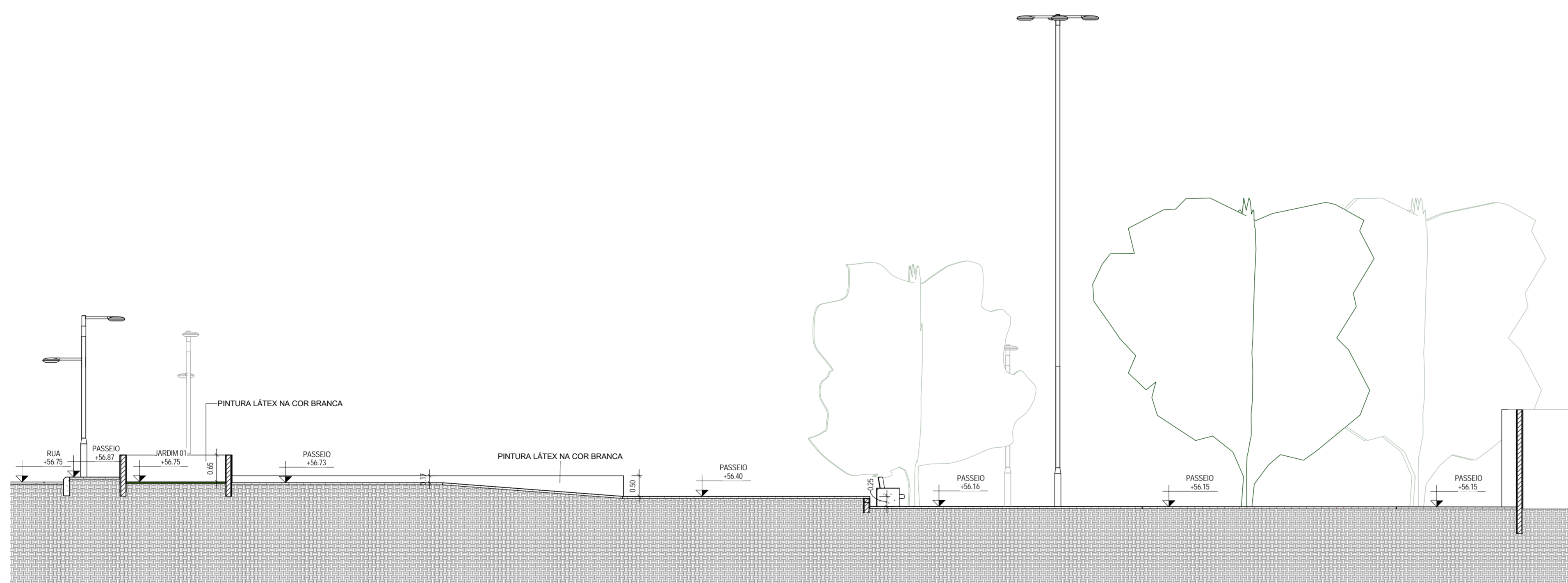
3 CORTE C-C 1:75
