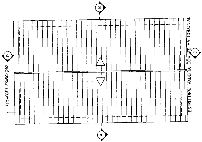
03 COBERTA VIVÊNCIA ESCALA: 1/100
