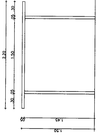
02 VISTA LATERAL ESCALA 1/30
