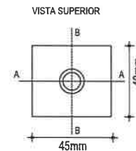
BRAQUETE ESCALA: 1/2
