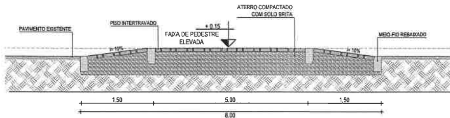
VISTA LATERAL SEM ESCALA
