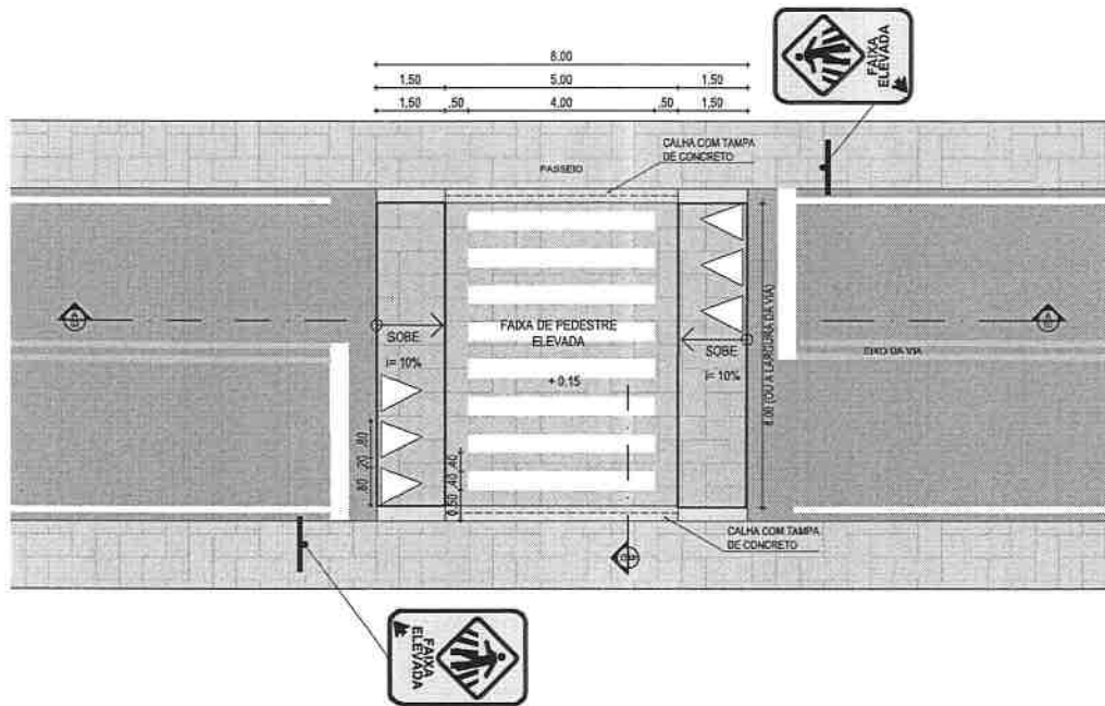
PLANTA BAIXA FAIXA ELEVADA SEM ESCALA
