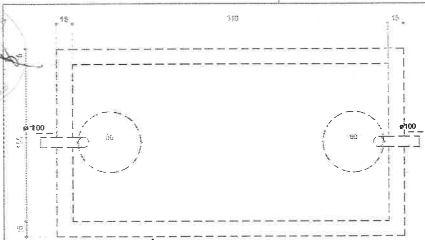
Tanque séptico - TÉRREO Planta baixa - ESC. 1:25
