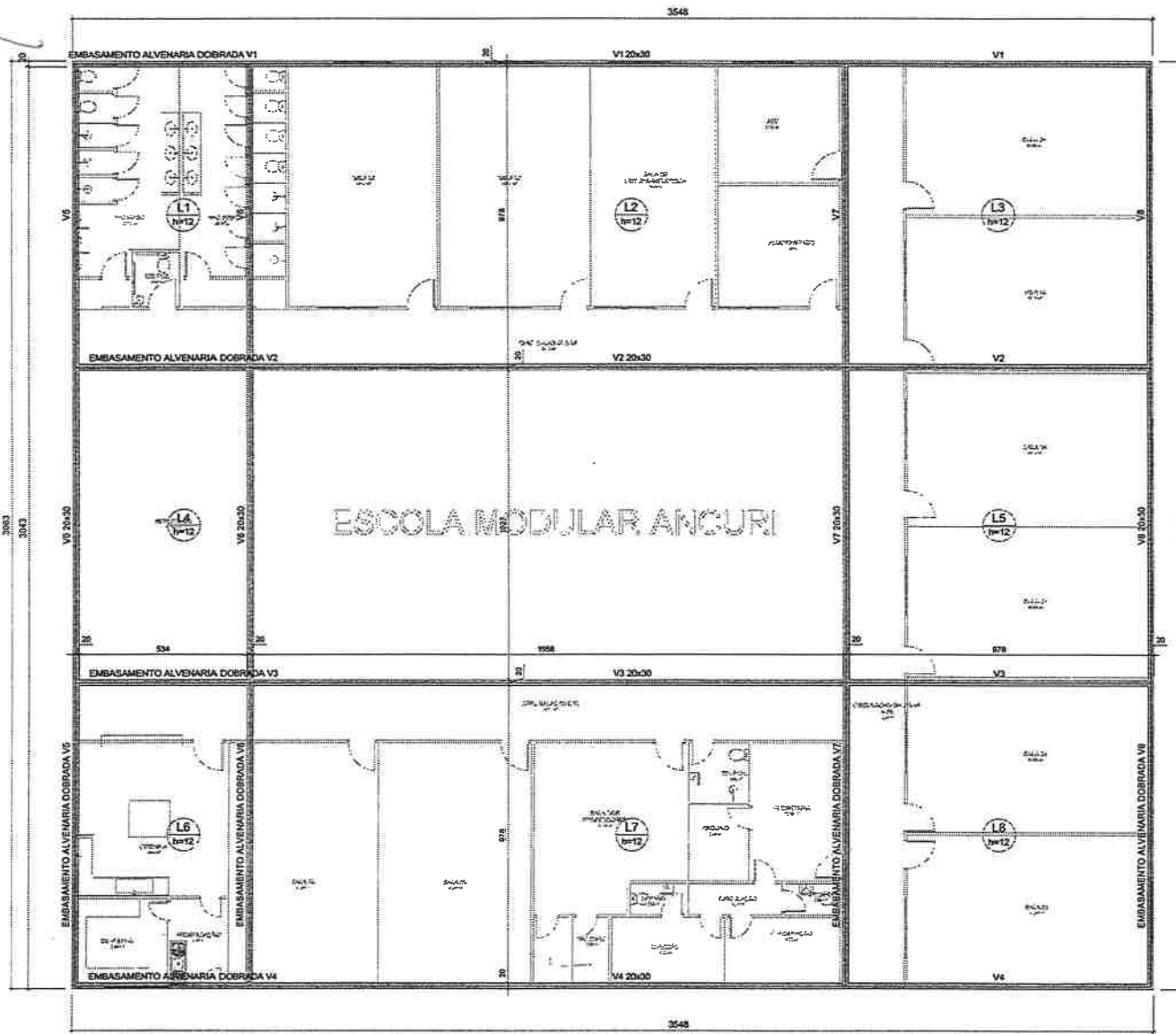
Forma do PISO - ESCOLA MODULAR ANCURI escala 1:150
