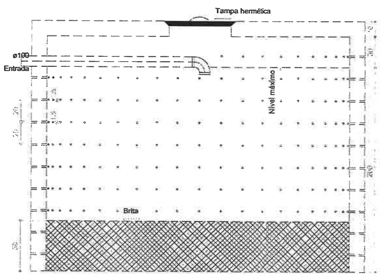
Sumidouro - TÉRREO Corte 1 - ESC. 1:25
