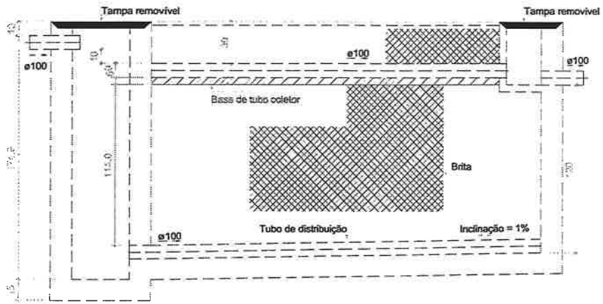
Filtro anaeróbio - TÉRREO Corte 1 - ESC. 1:25
