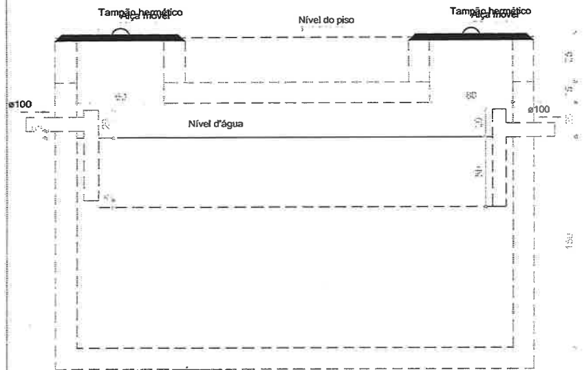
Tanque séptico - TÉRREO Corte 1 - ESC. 1:25
