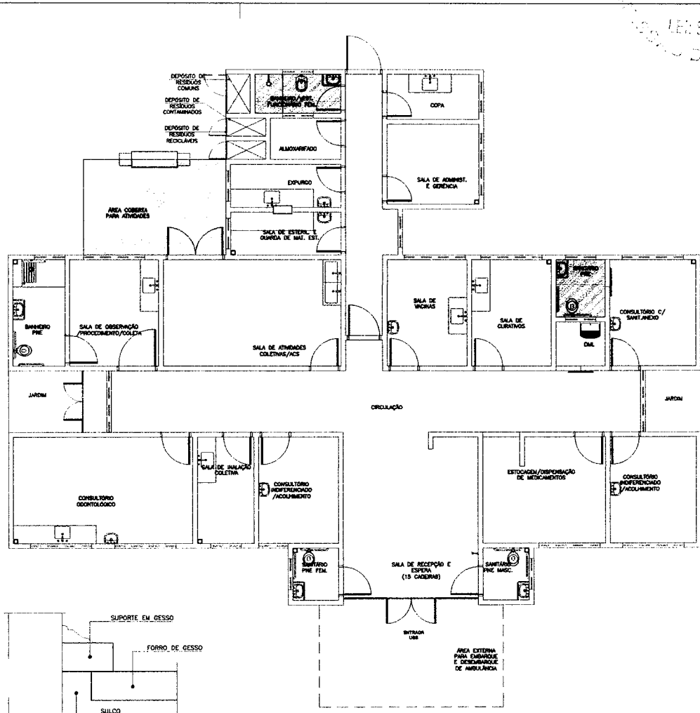
Planta Baixa Acabamento Teto Nível: D.00 Esc.: 1:100
