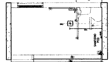
-Planta Bases 1:20 1991 1991
