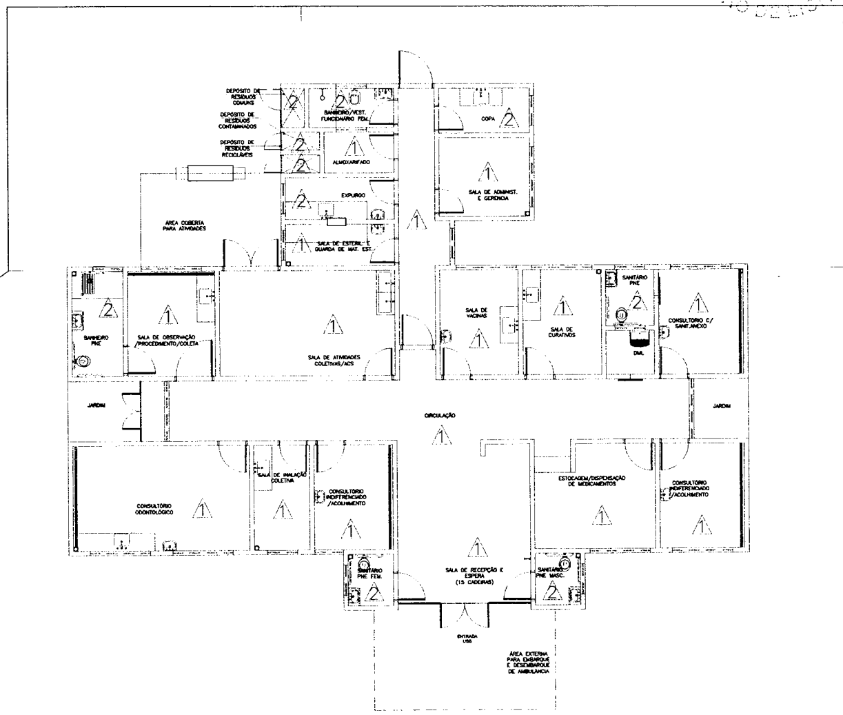
Planta Baixa Acabamento Parede Nível: 0.00 Esc.: 1:100
