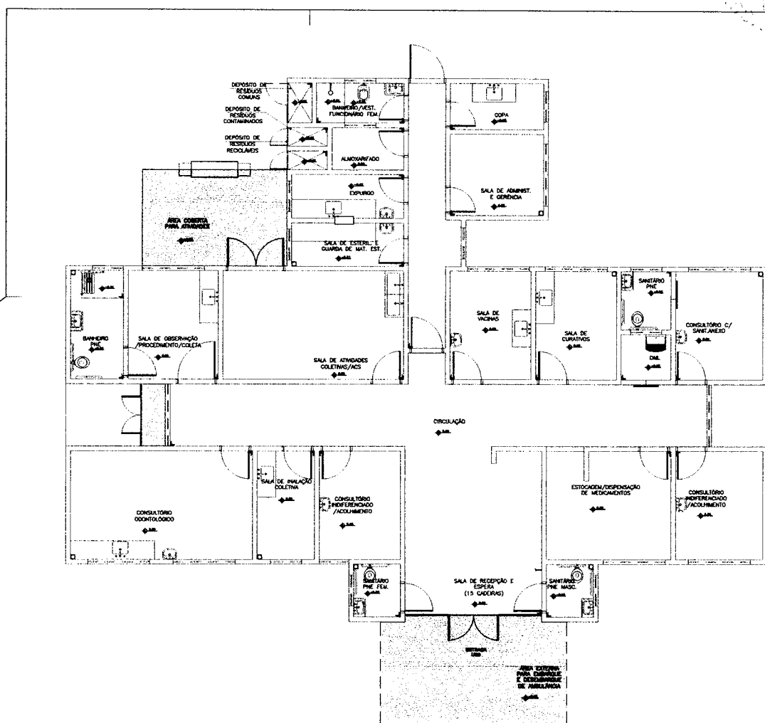
Planta Baixa Acabamento Piso Nível: 0,00 Esc.: 1:100
