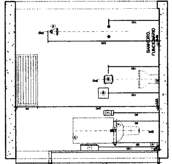
-Sección AA' 1:20 1991 1991
