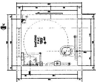
-Planta Bases 1:20 1991 1991
