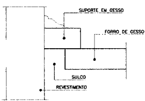
Detalhe Junta de Dilatação Sem Escala
